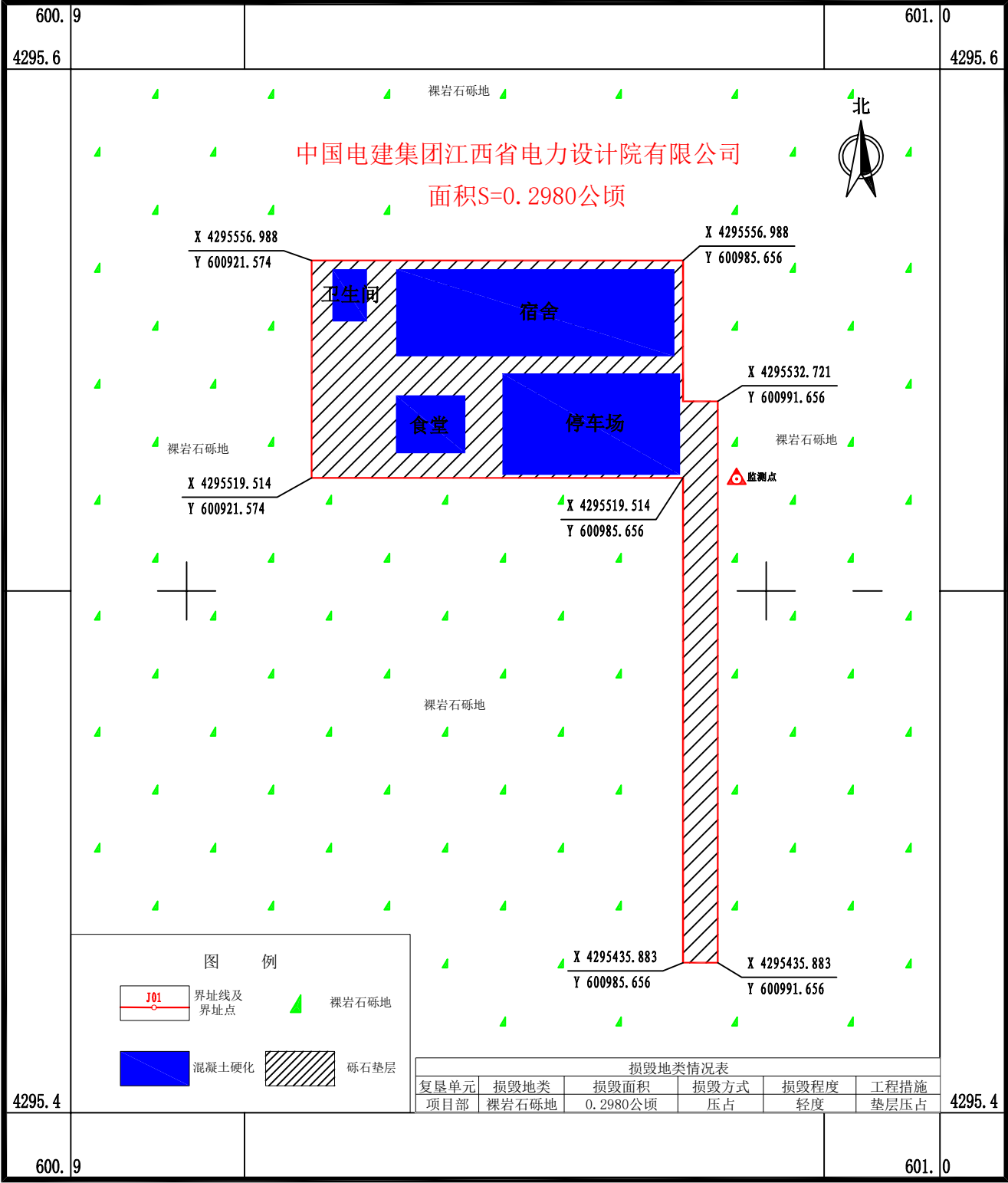
塔里木油田巴州若羌100万千瓦光伏发电项目升压储能站标(工人生活区)临时用地土地损毁预测图
