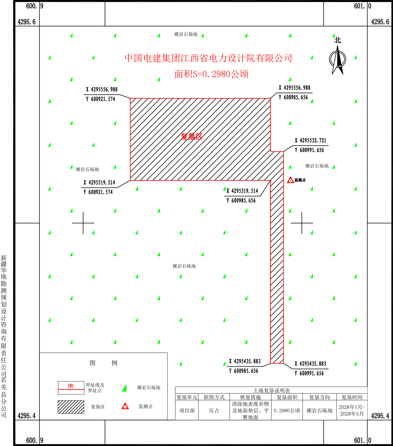
塔里木油田巴州若羌100万千瓦光伏发电项目升压储能站标(工人生活区)临时用地土地复垦图
