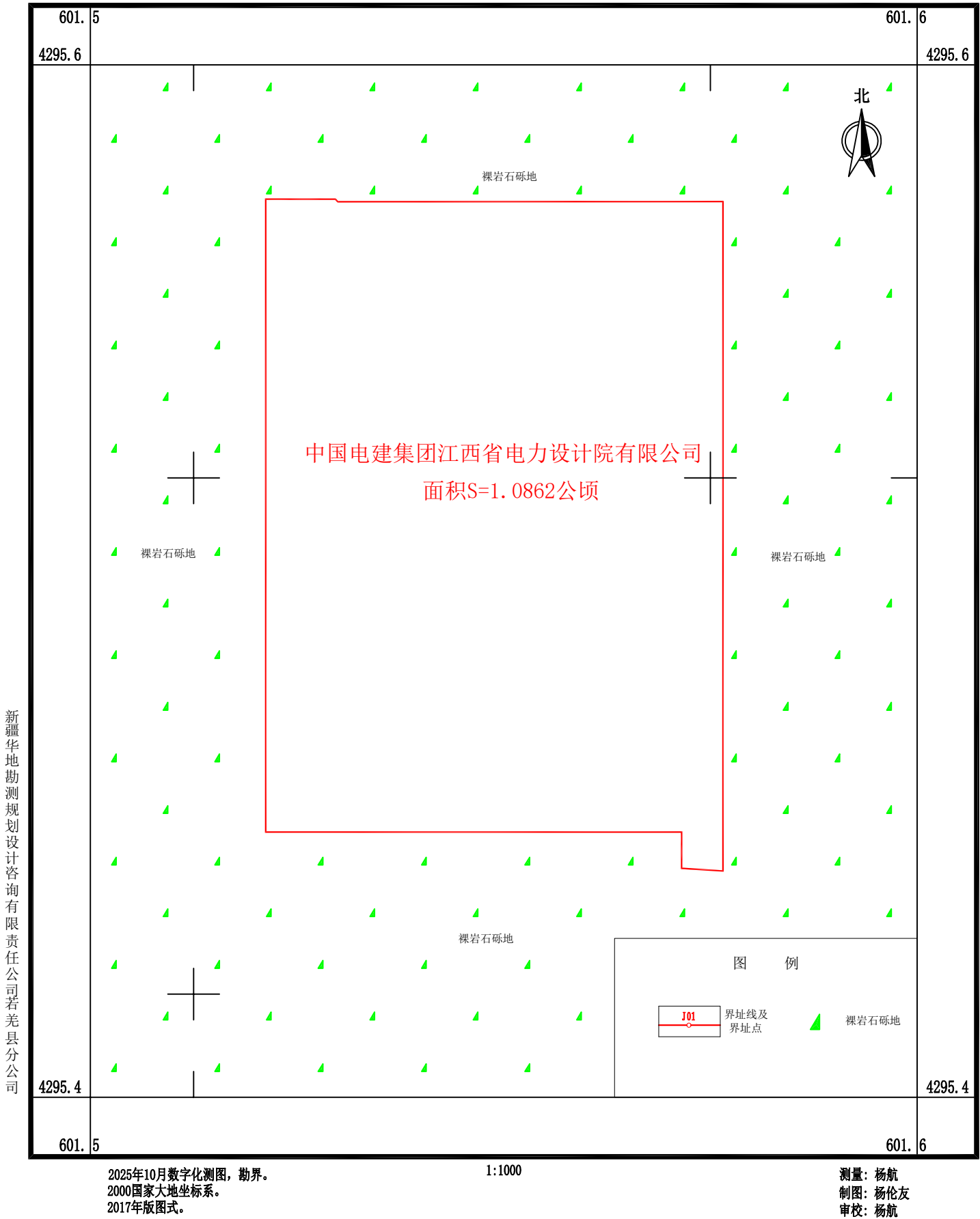
塔里木油田巴州若羌100万千瓦光伏发电项目升压汇集站和储能站EPC总承包项目部临时用地土地利用现状图
