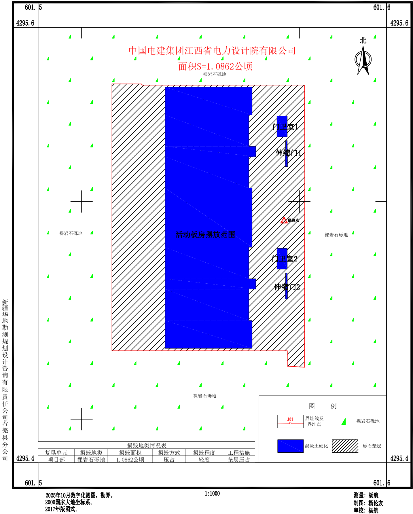
塔里木油田巴州若羌100万千瓦光伏发电项目升压汇集站和储能站EPC总承包项目部临时用地土地损毁预测图
